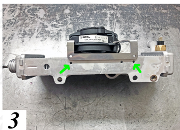
Fig.3-4 Fissare con rivetti negli appositi buchi già presenti sui radiatori/ Fig.3-4 Secure with rivets in the appropriate holes already present on the radiators
