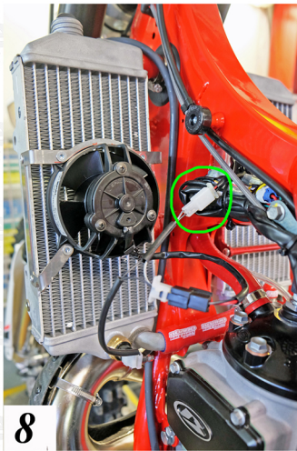
Fig. 8 montare il radiatore sulla moto collegandolo all'impianto elettrico principale/ Fig. 8 mount the radiator on the motorcycle by connecting it to the main electrical system
