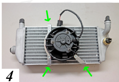
Fig.3-4 Fissare con rivetti negli appositi buchi già presenti sui radiatori/ Fig.3-4 Secure with rivets in the appropriate holes already present on the radiators
