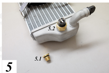
Fig. 5 Sostituire il tappo (5.1) con il bulbo in dotazione (5.2)/ Fig. 5 Replace the cap (5.1) with the bulb supplied (5.2)
